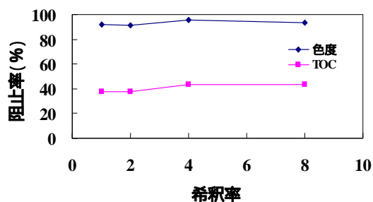
図13 希釈による色度及びTOC阻止率への効果 膜の分画分子量：1,000
