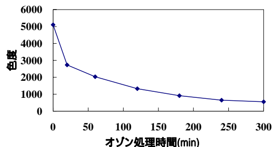
図14 オゾン処理による膜透過液の脱色
