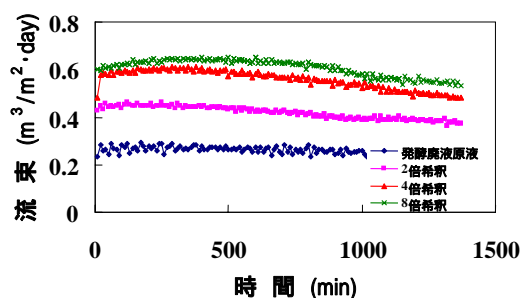
図12 希釈による流束への効果 膜の分画分子量：1,000
