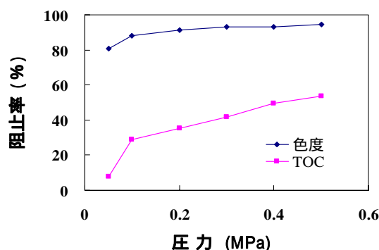
図10 圧力と色度及び TOC 阻止率の関係 膜の分画分子量 : 1,000
