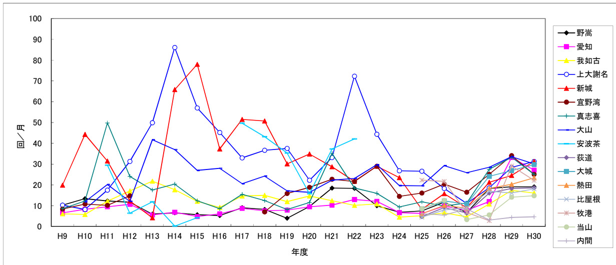
図F3-2 飛行等制限時間帯(22:00～6:00)における騒音発生回数の年度推移 [全測定局]
