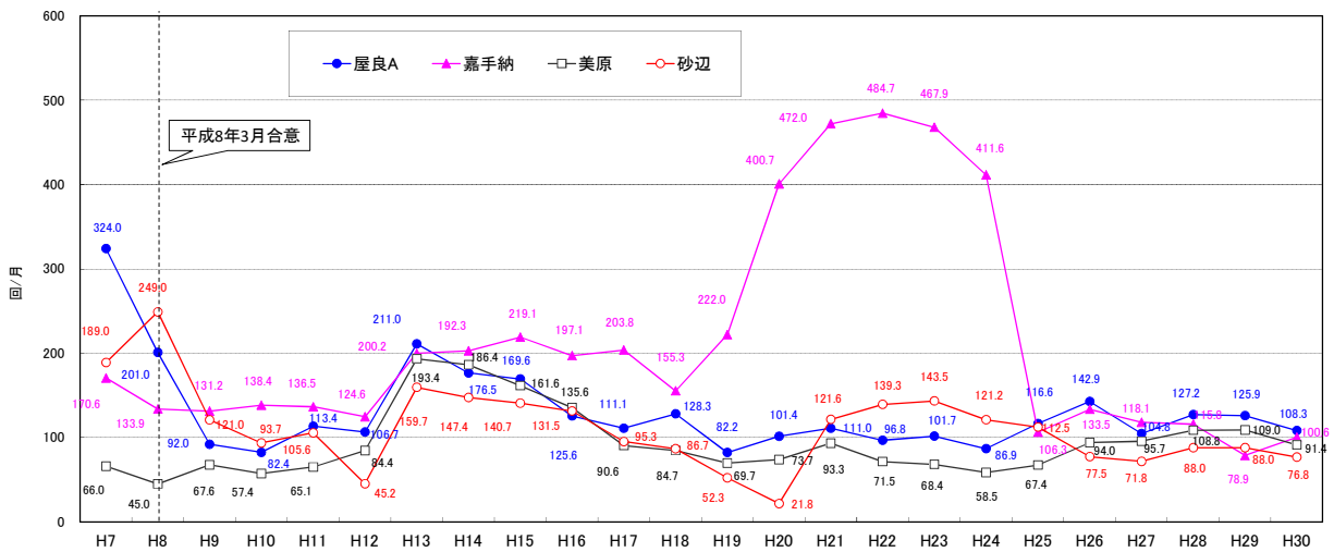
図K2-2 航空機騒音規制措置合意前後の航空機騒音発生状況 (騒音発生回数の年度別推移、夜間(22時)～早朝(7時))
