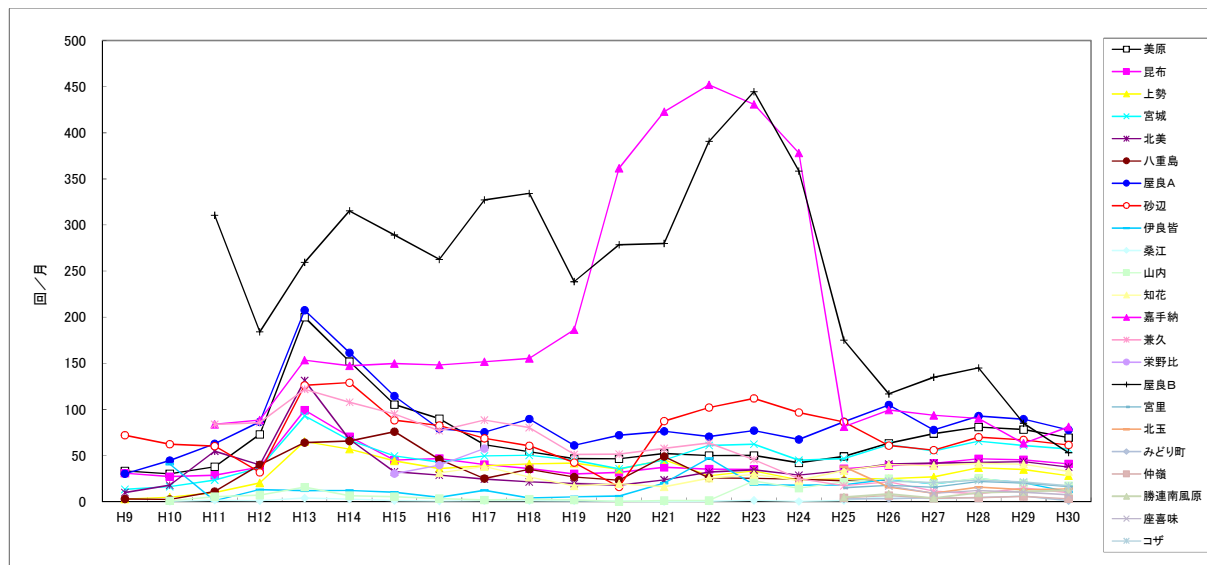
図K3-2 飛行等制限時間帯(22:00~6:00)における騒音発生回数の年度推移 [全測定局]
