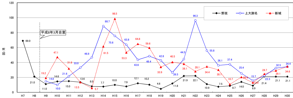
図F2-2 航空機騒音規制措置合意前後の航空機騒音発生状況 (騒音発生回数の年度別推移、夜間(22時)～早朝(7時))
