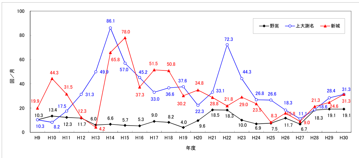
図F3 飛行等制限時間帯(22:00～6:00)における騒音発生回数の年度推移
