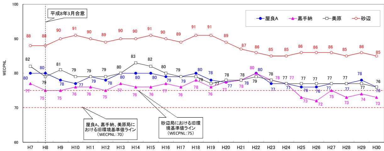
図K2 航空機騒音規制措置合意前後の航空機騒音発生状況 (WECPNLの年度別推移)
