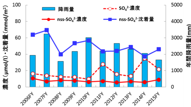
図 2. SO 4 2- (wet) 濃度, nss-SO 4 2- (wet) 濃度および nss-SO 4 2- (wet) 沈着量の年平均値と年間降雨量の経年変動. SO 4 2- (wet) 濃度は海塩の影響により大きく変動し, nss-SO 4 2- (wet) 濃度はほぼ横ばいで推移した. nss-SO 4 2- (wet) 沈着量は年間降雨量の増減と類似した挙動を示しながら, やや減少傾向を示した.
