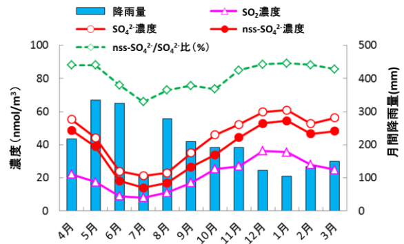
図 5. 乾性沈着の月平均値、 nss-SO_4^{2-}(p)/SO_4^{2-}(p) 比および月間降雨量の経月変動。 nss-SO_4^{2-}(p) 濃度などはいずれも春季および冬季に高くなる、同様の挙動を示し、 nss-SO_4^{2-}(p)/SO_4^{2-}(p) 比は 7-10 月に低くなっていた。
