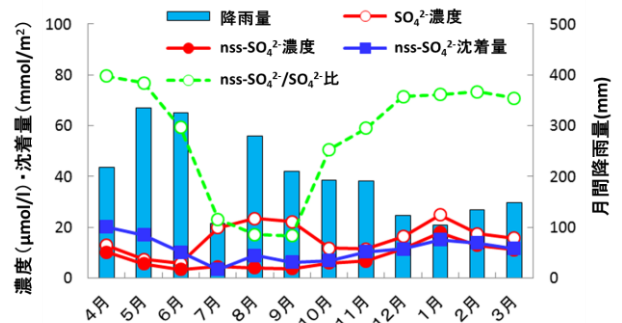
図 4. 湿性沈着の月平均値と月間降雨量の経月変動. SO 4 2- (wet) 濃度は 8 月および 1 月にピークとなる 2 山型を, nss-SO 4 2- (wet) 濃度は 1 月にピークとなる 1 山型を, nss-SO 4 2- (wet) 沈着量は 4 月および 1 月にピークとなる 2 山型を示した.
