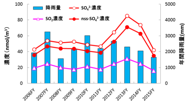
図 3. SO 4 2- (p) 濃度, nss-SO 4 2- (p) 濃度および SO 2 (g) 濃度の年平均値と年間降雨量の経年変動. SO 4 2- (p) 濃度, nss-SO 4 2- (p) 濃度および SO 2 (g) 濃度は同様の挙動を示し, 年間降雨量との相関は認められなかった.
