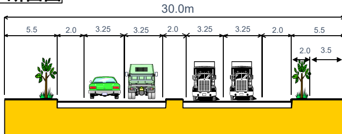
標準断面図
