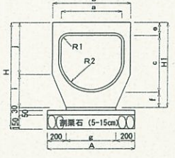
DO管
