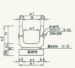
U字溝
