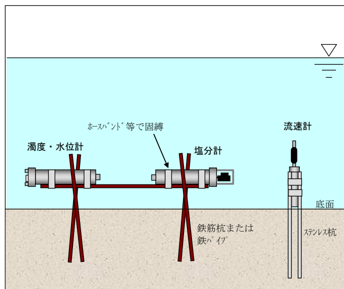
図 2.7.5 機器の設置方法 (機器の種類は地点により異なる)
