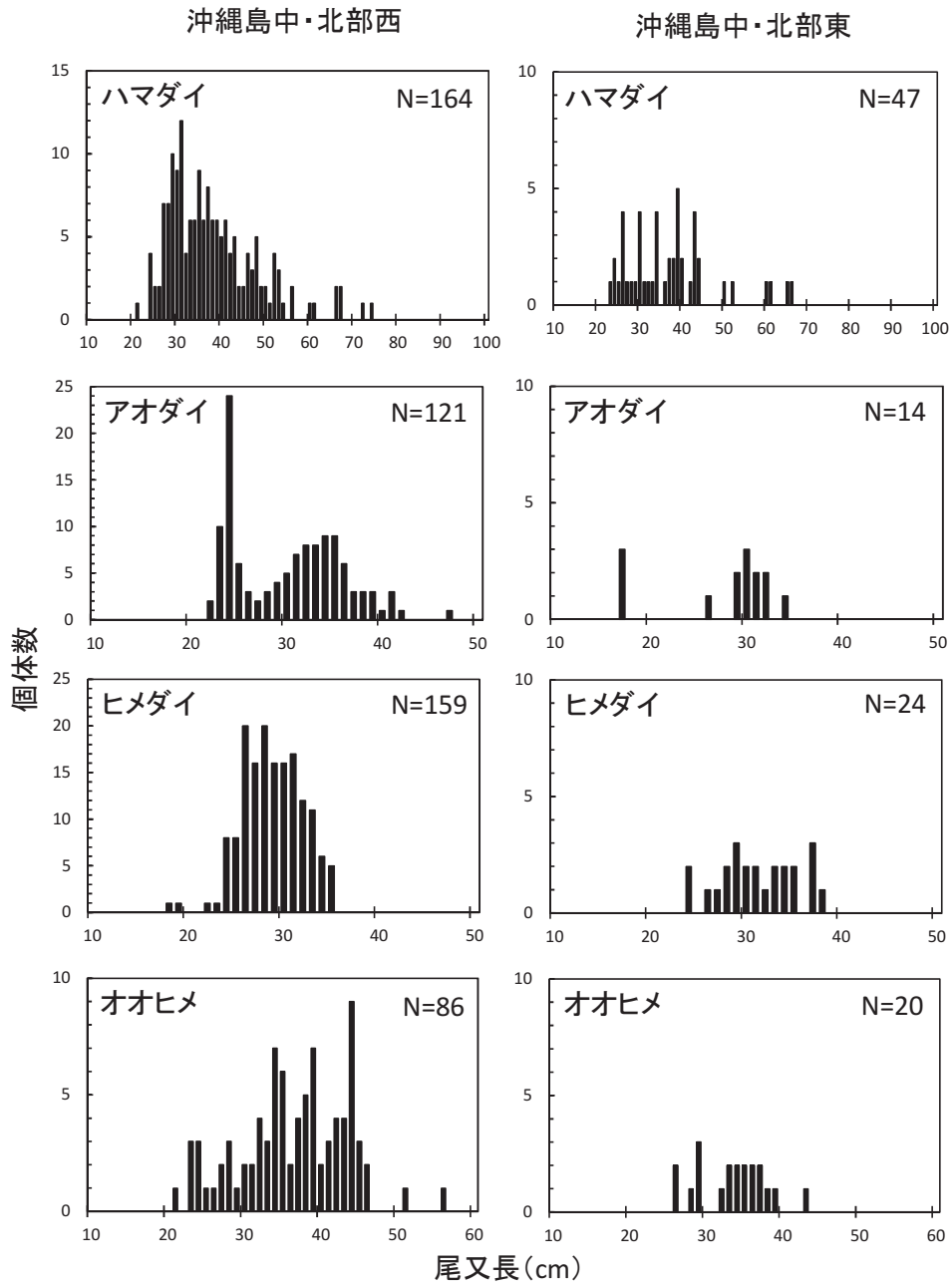
図 中・北部地域のセリ市場に水揚げされたマチ類 4 種の尾又長組成
