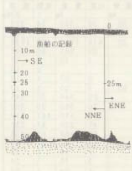
4 魚礁の設置状況 a 魚礁設置断面(魚探記録)
