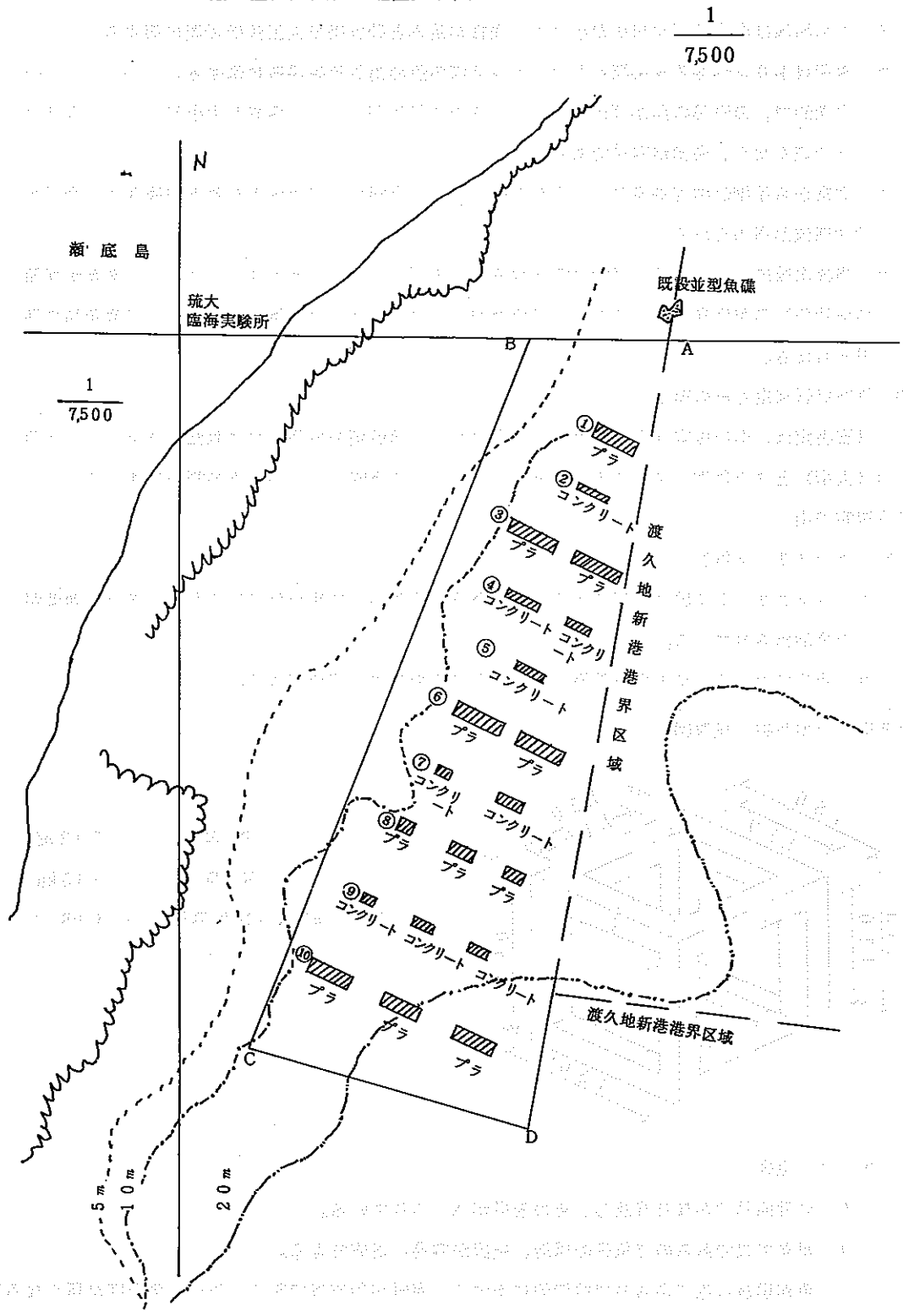
第7図 人工魚礁設置位置拡大図及び配置見取図
