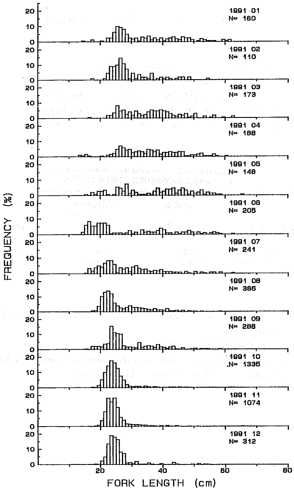
図 14 調査海域から名護漁協に水揚げされたハマフエフキの月別尾叉長組成
