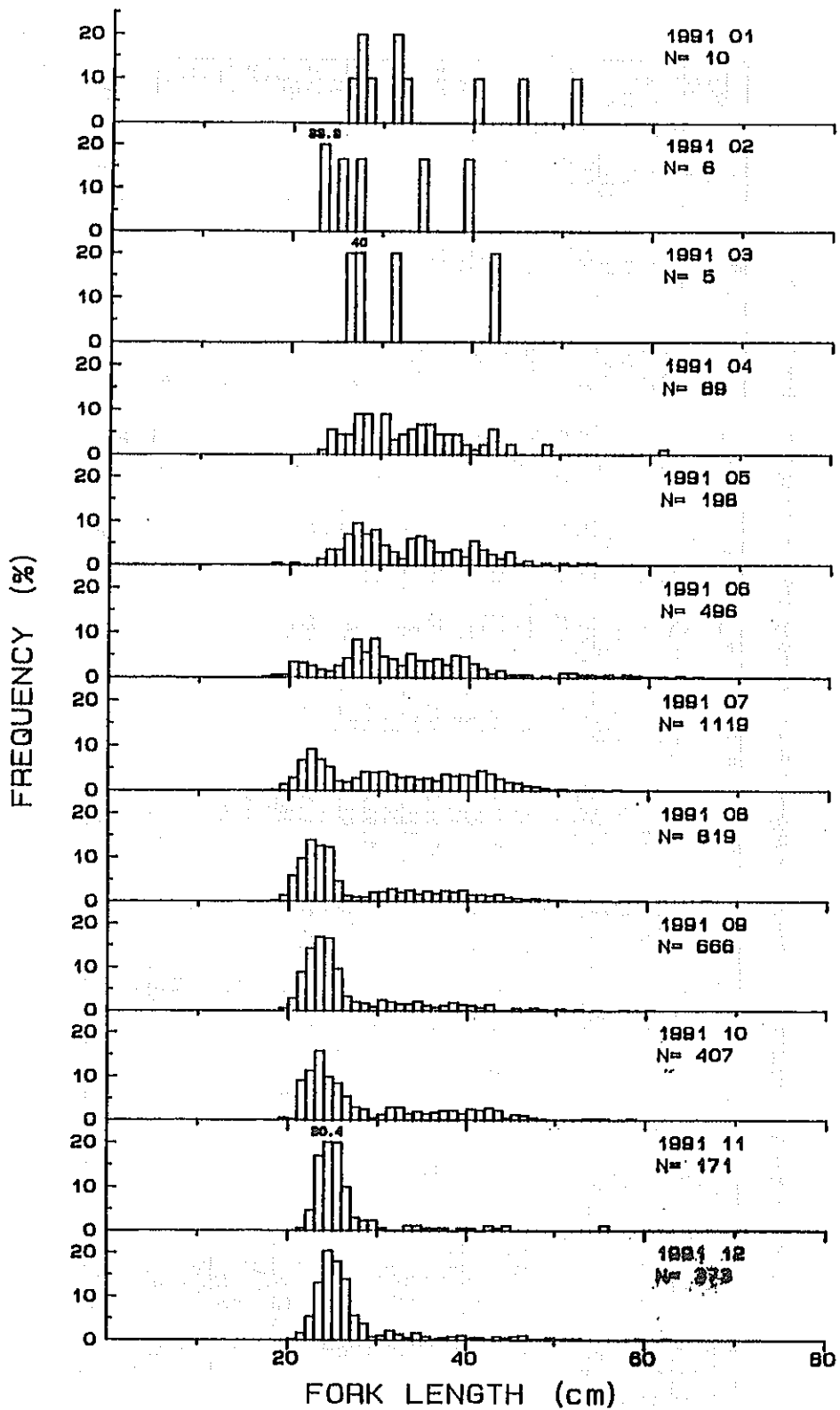
図 15 調査海域から国頭漁協に水揚げされたハマフエフキの月別尾叉長組成
