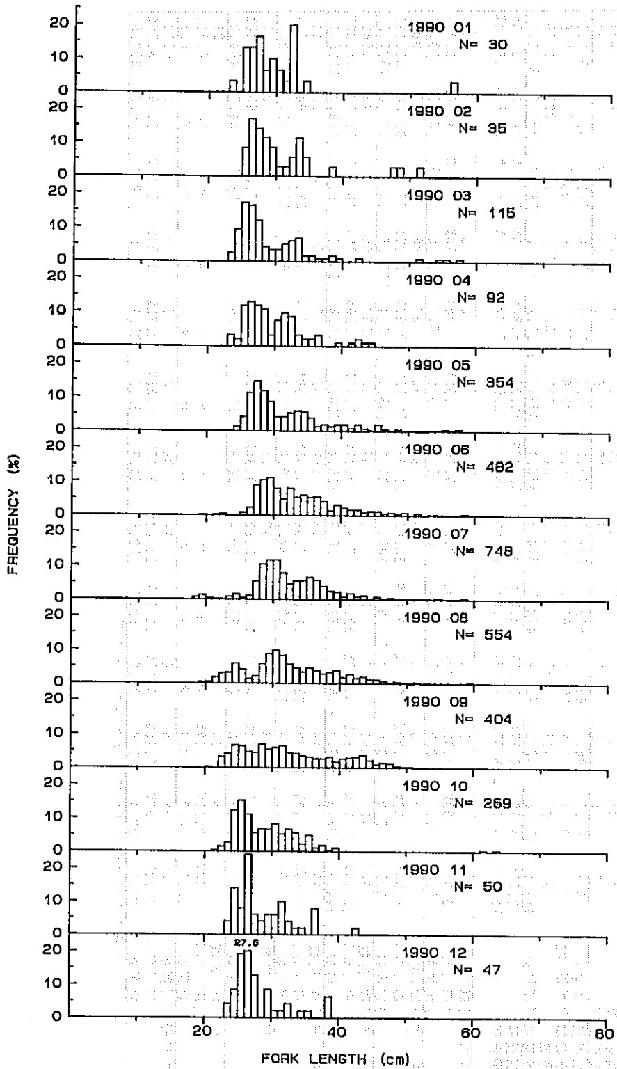
図12 調査海域から国頭漁協に水揚げされたハマフエフキの月別尾叉長組成
