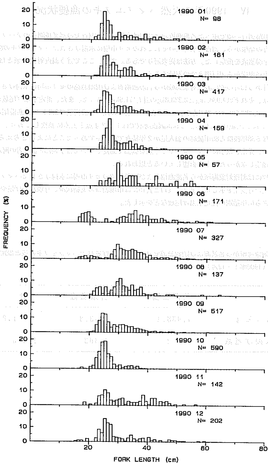
図11 調査海域から名護漁協に水揚げされたハマフエフキの月別尾又長組成
