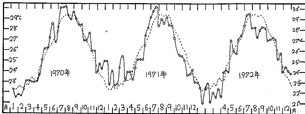
図9 魚釣島 (25°-45'N 123°-30'E) の水温変化
