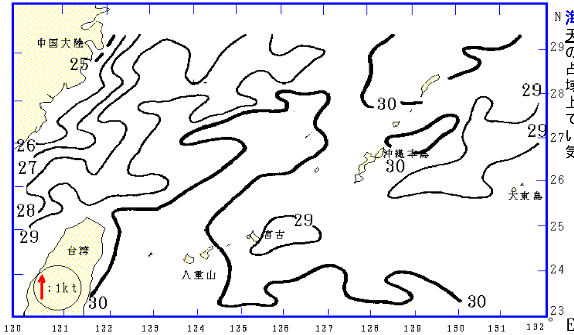
図1 表面水温分布図(1998年8月25日)
