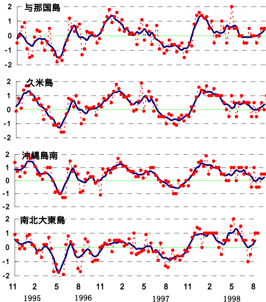
図2 沖縄近海における表面水温偏差(目盛りは旬)
