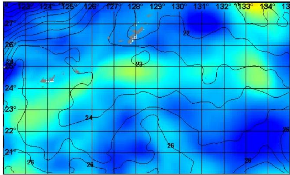
図1. 海況案内人による表面水温(等温度線)・海面高度分布(塗り分け)図(2023年3月31日)
