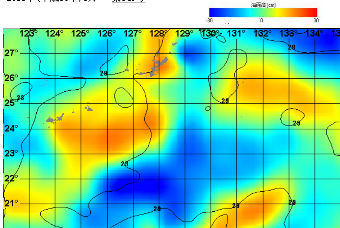
図1. 海況案内人による表面水温(等温度線)・海面高度分布(塗り分け)図(2018年8月31日)
