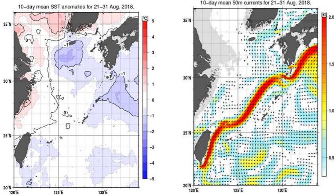
図2. 2018年8月下旬海面水温偏差図(左)及び海流図(気象庁HPより)
