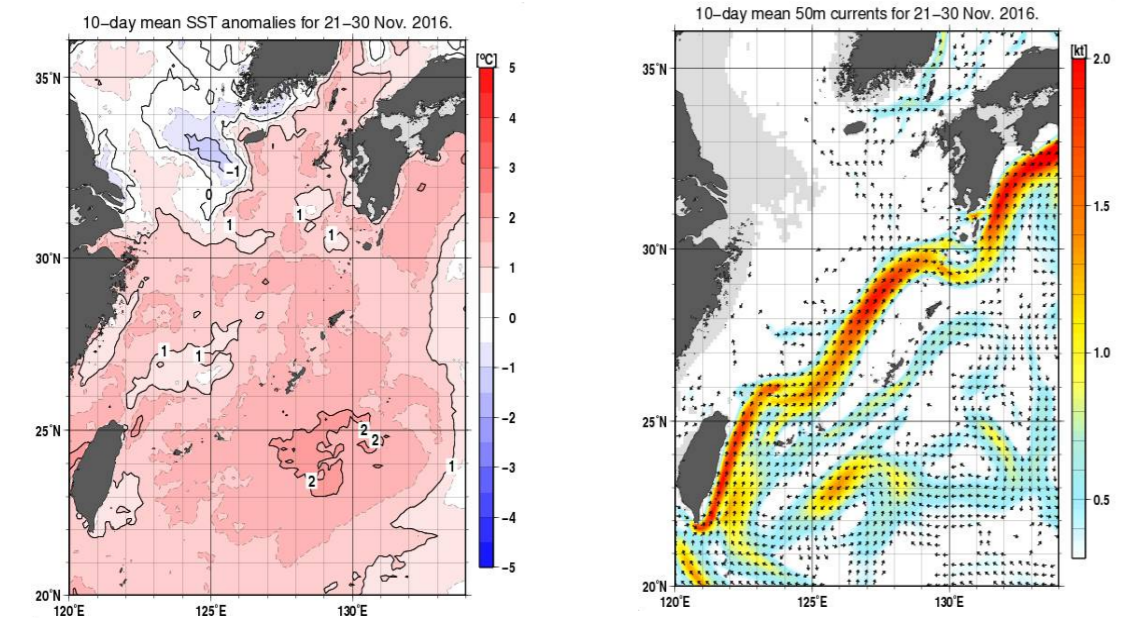
図2. 2016年11月下旬海面水温偏差図(左)及び海流図(気象庁HPより)
