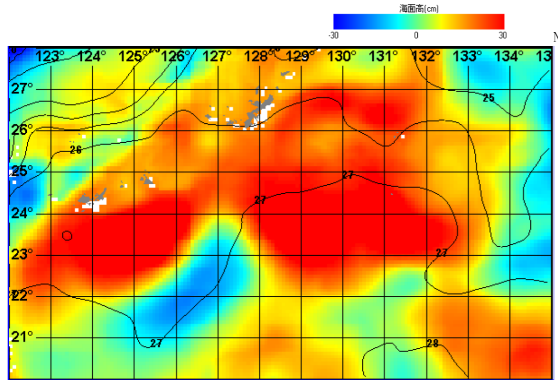
図1. 海況案内人による表面水温(等温度線)・海面高度分布(塗り分け)図(2016年11月30日)
