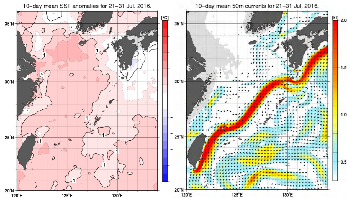
図2. 2016年7月下旬海面水温偏差図(左)及び海流図(気象庁HPより)
