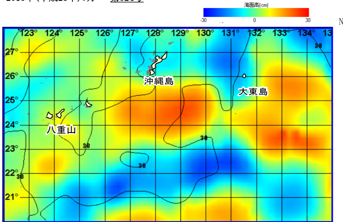
図1. 海況案内人による表面水温(等温度線)・海面高度分布(塗り分け)図(2016年7月19日)
