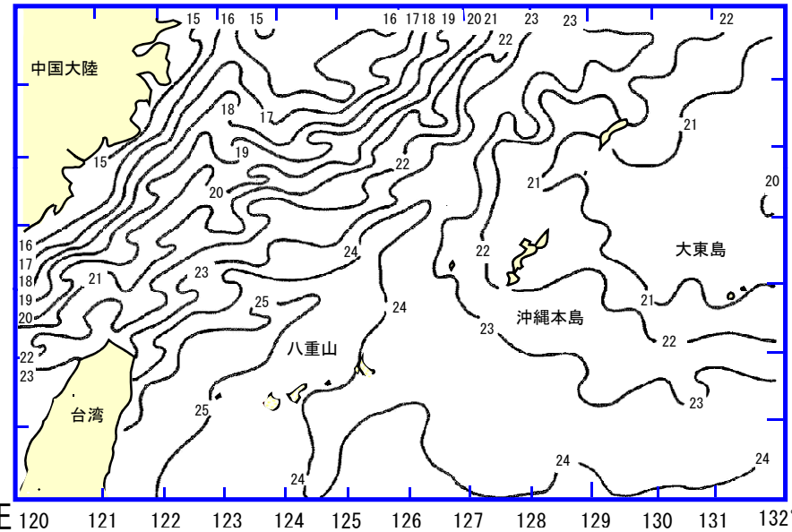
図1. 表面水温分布図(2007年4月17日) 資料: 東シナ海海況速報(漁業情報サービスセンター)
