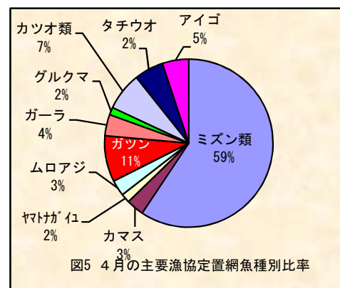
図5 4月の主要漁協定置網魚種別比率
