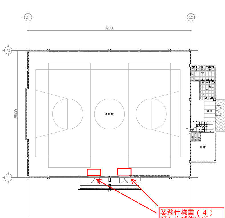
1F平面図 1/300
