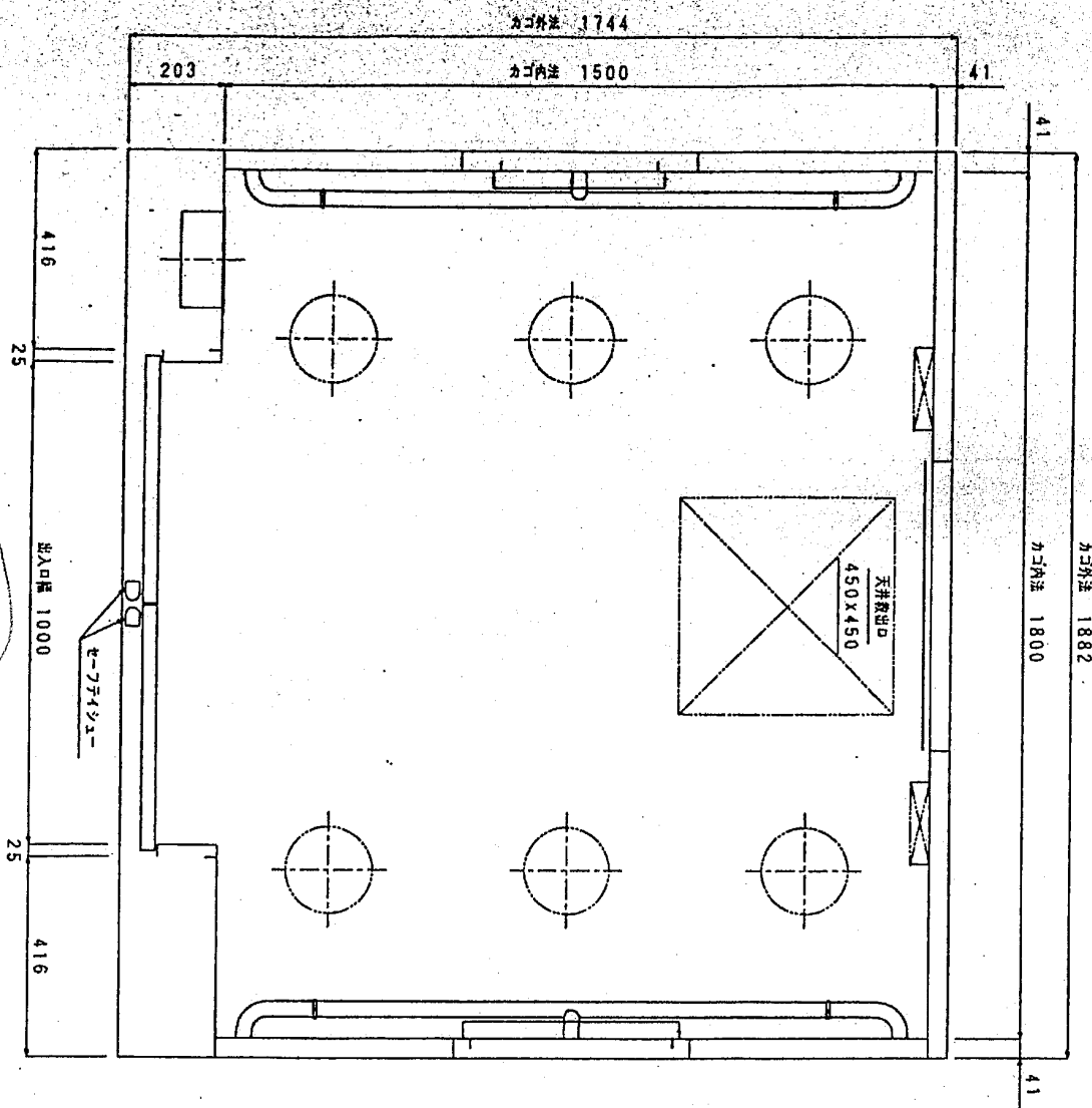
平面図
