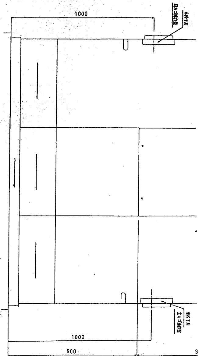
背面図
