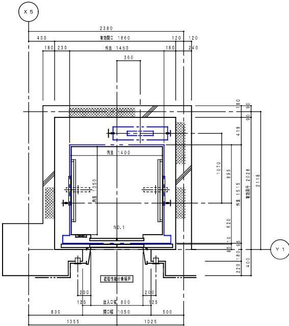
2.3 階 昇降路平面図 (1:40)
