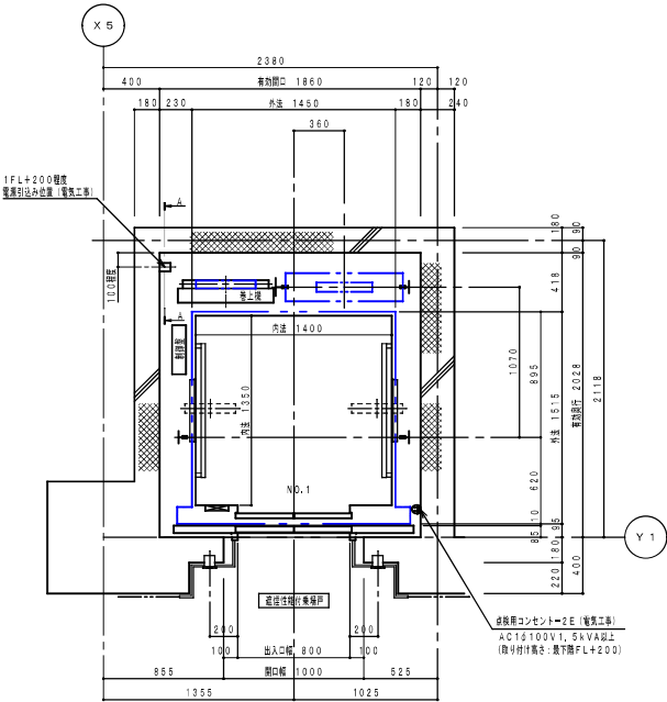
1 階 昇降路平面図 (1:40)
