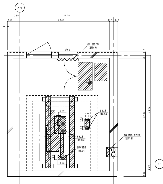
机械室平面图 (1:20)
