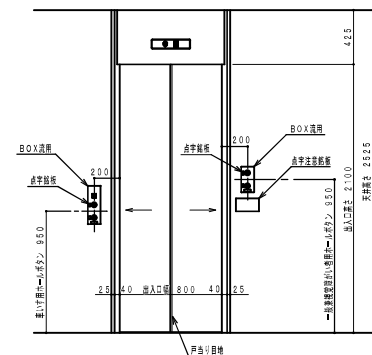
2階 出入口正面及断面図 (1:20)
