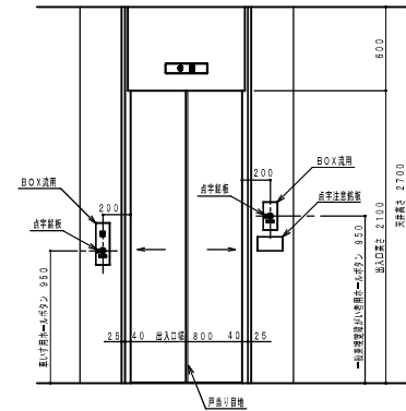
3階 出入口正面及断面図 (1:20)
