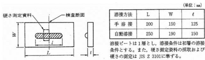
図 3 - 3 - 4 最高硬さ試験, 試験体形状及び試験片採取位置
