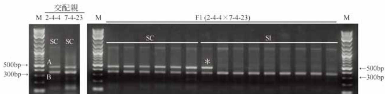
図3 自家和合性特異的な SC22360 から変換した DNA マーカー SC_In/Del
