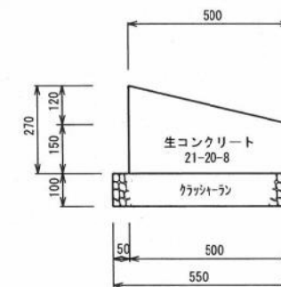
水兼農道側壁(B型)
