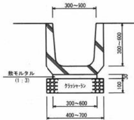
U字溝標準断面図
