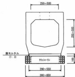
管渠型側溝標準断面図
