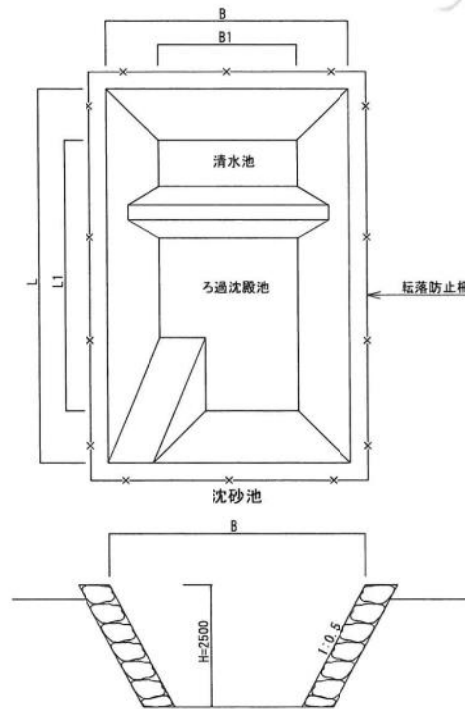
浸透池・沈砂池標準断面図
