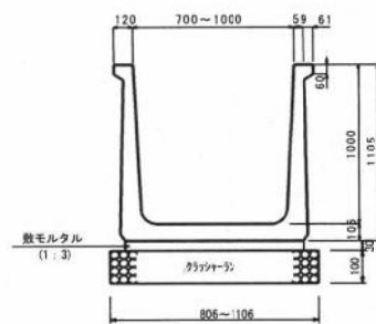
フリューム標準断面図
