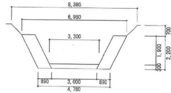
C型排水路
