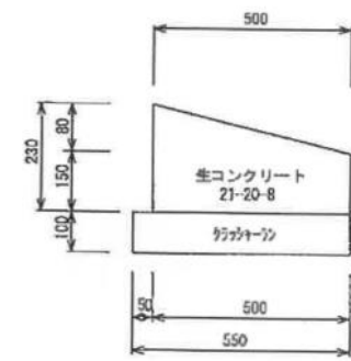
水兼農道側壁(A型)
