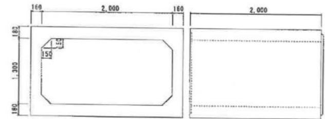
RCボックスカルバート(横断溝K-2) B2000×H1300×L2000
