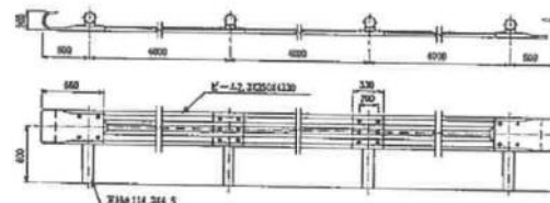
ガードレール Gr-C-4E
