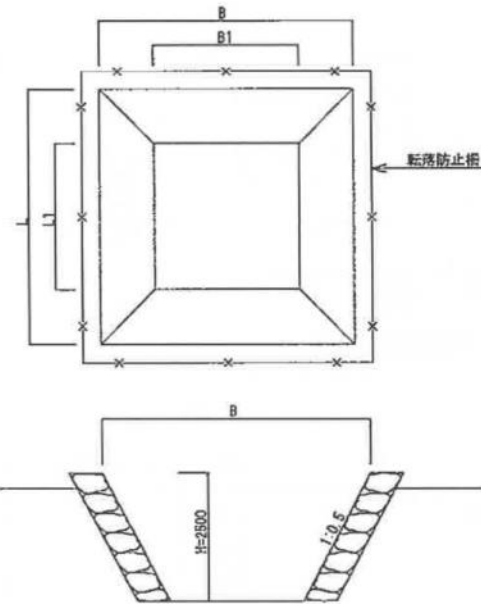
浸透池標準断面図
