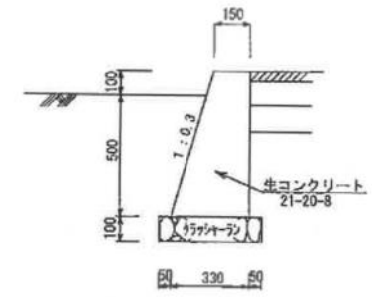
鍬止工
