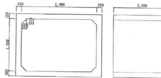
RCボックスカルバート(横断溝K-1) B2900×H1900×L2000
