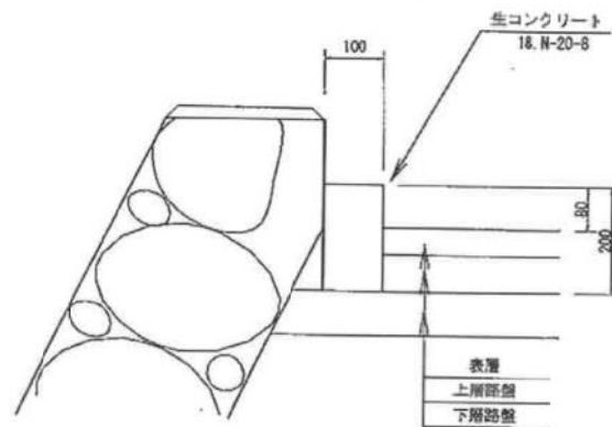
舗装止工
