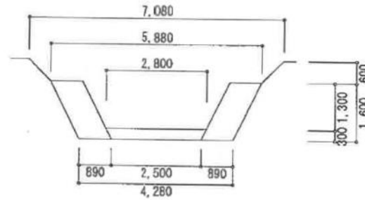
B型排水路
