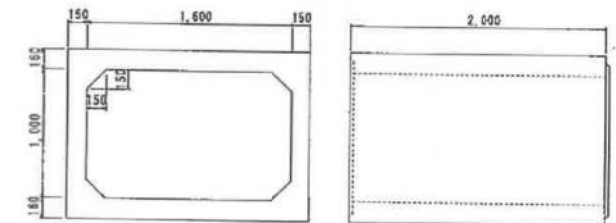
RCボックスカルバート(横断溝S-1) B1800×H1000×L2000
