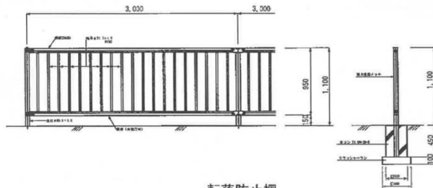
転落防止柵
