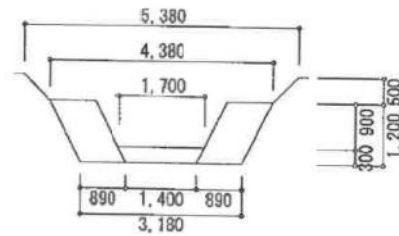
支線排水路
