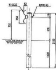
ガードレール Gr-C-4E
