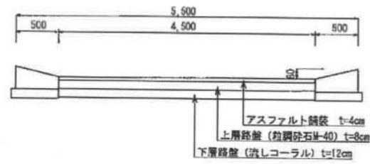
水兼農道標準断面図
