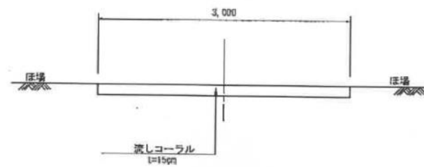
耕作道標準断面図
