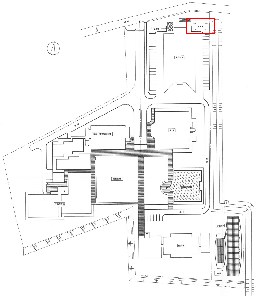
配置図 S=1:500
