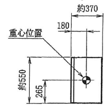
インバータ 搬入質量 約110Kg(ETI-20)
