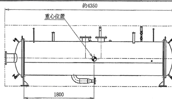
蒸発器ユニット 搬入質量 約2720Kg
