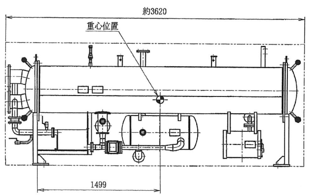
凝縮器ユニット 搬入質量 約1420Kg
