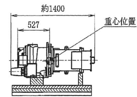
圧縮機B・電動機Bユニット 搬入質量 約870Kg
