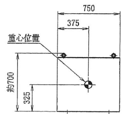
操作盤 搬入質量 約60Kg
