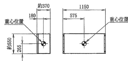
インバータ 搬入質量 約110Kg x 2個 (ETI-40)
