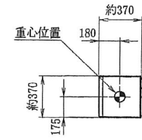
インバータ 搬入質量 約90Kg(ETI-15)
