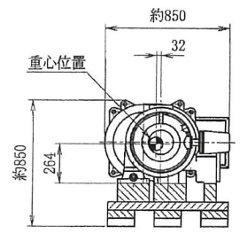
圧縮機・電動機ユニット 搬入質量 約870Kg
