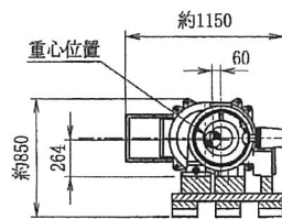
圧縮機A・電動機Aユニット 搬入質量 約870Kg
