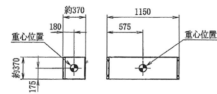
インバータ 搬入質量 約90Kg x 2個 (ETI-30)
