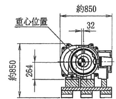
圧縮機B・電動機Bユニット 搬入質量 約870Kg
