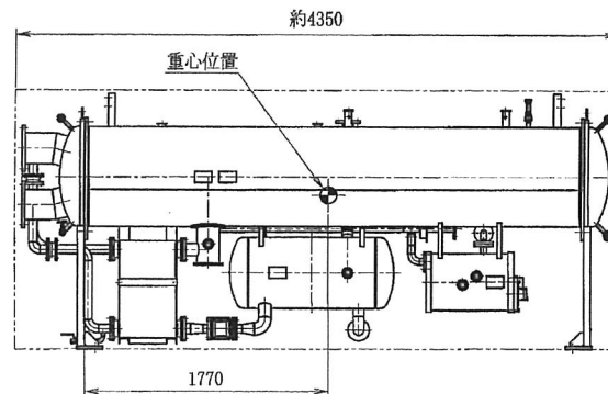
凝縮器ユニット 搬入質量 約2490Kg
