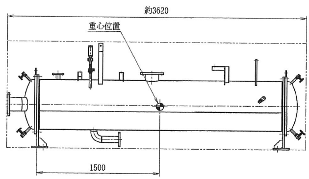
蒸発器ユニット 搬入質量 約1350Kg
