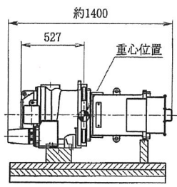
圧縮機・電動機ユニット 搬入質量 約870Kg
