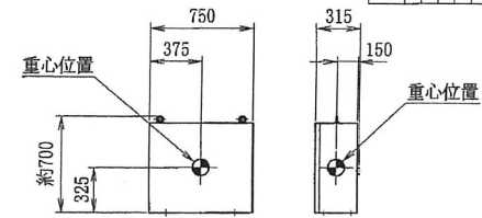
操作盤 搬入質量 約60Kg
