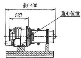
圧縮機A・電動機Aユニット 搬入質量 約870Kg
