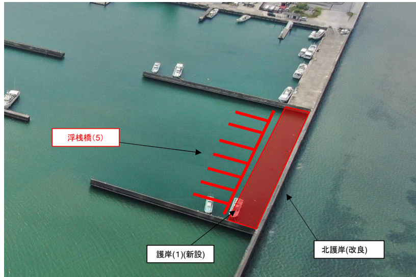
浮棧橋（5）施工予定箇所
