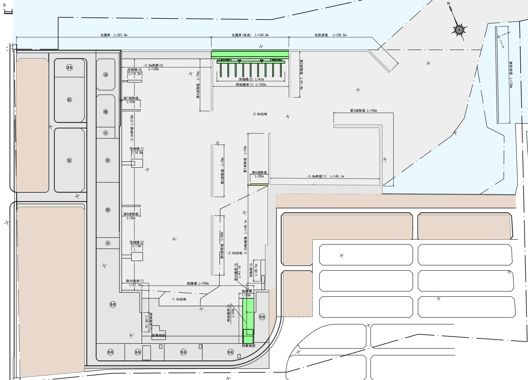
漁 港 区 域 図
