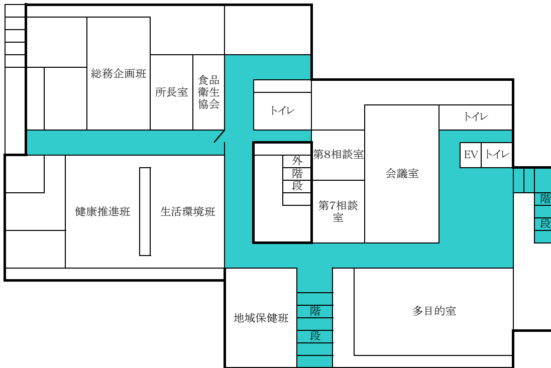
1階平面図
