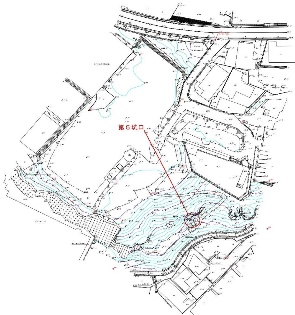
第5坑口周辺現況平面図
