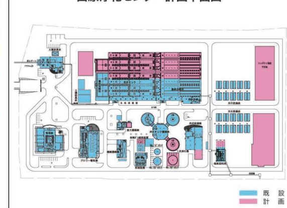
西原浄化センター計画平面図
