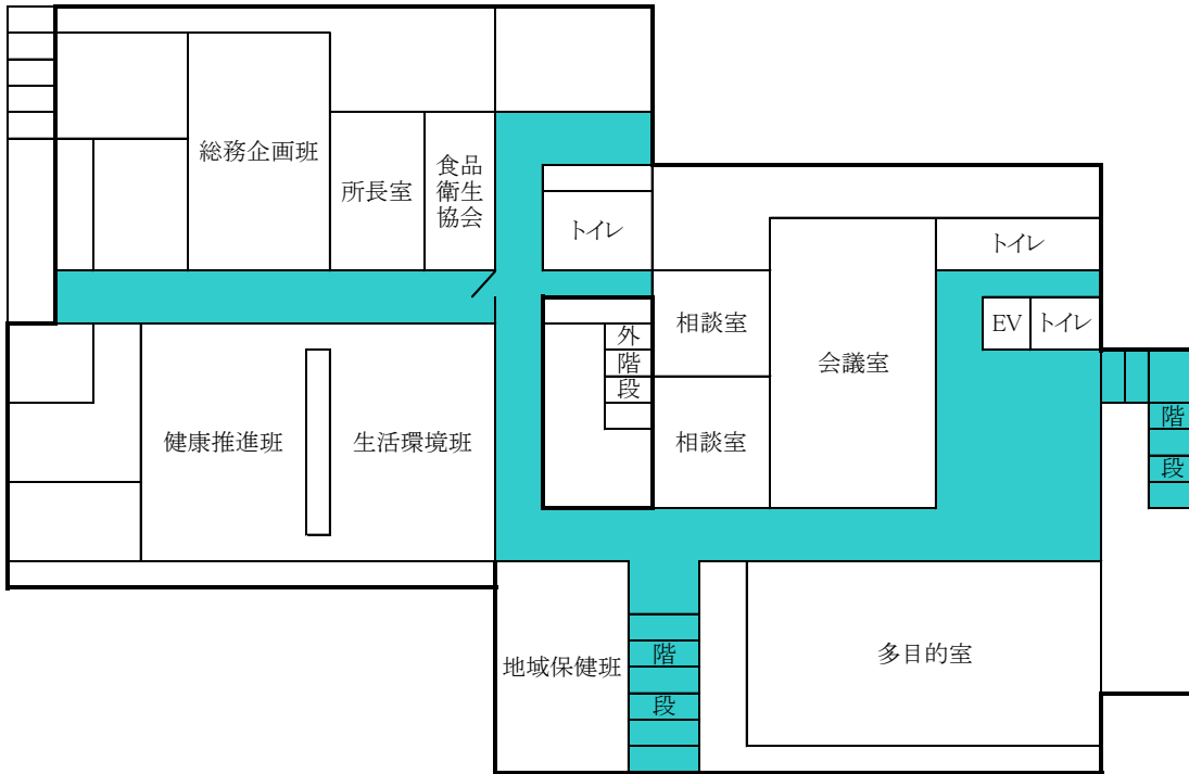
1階平面図
