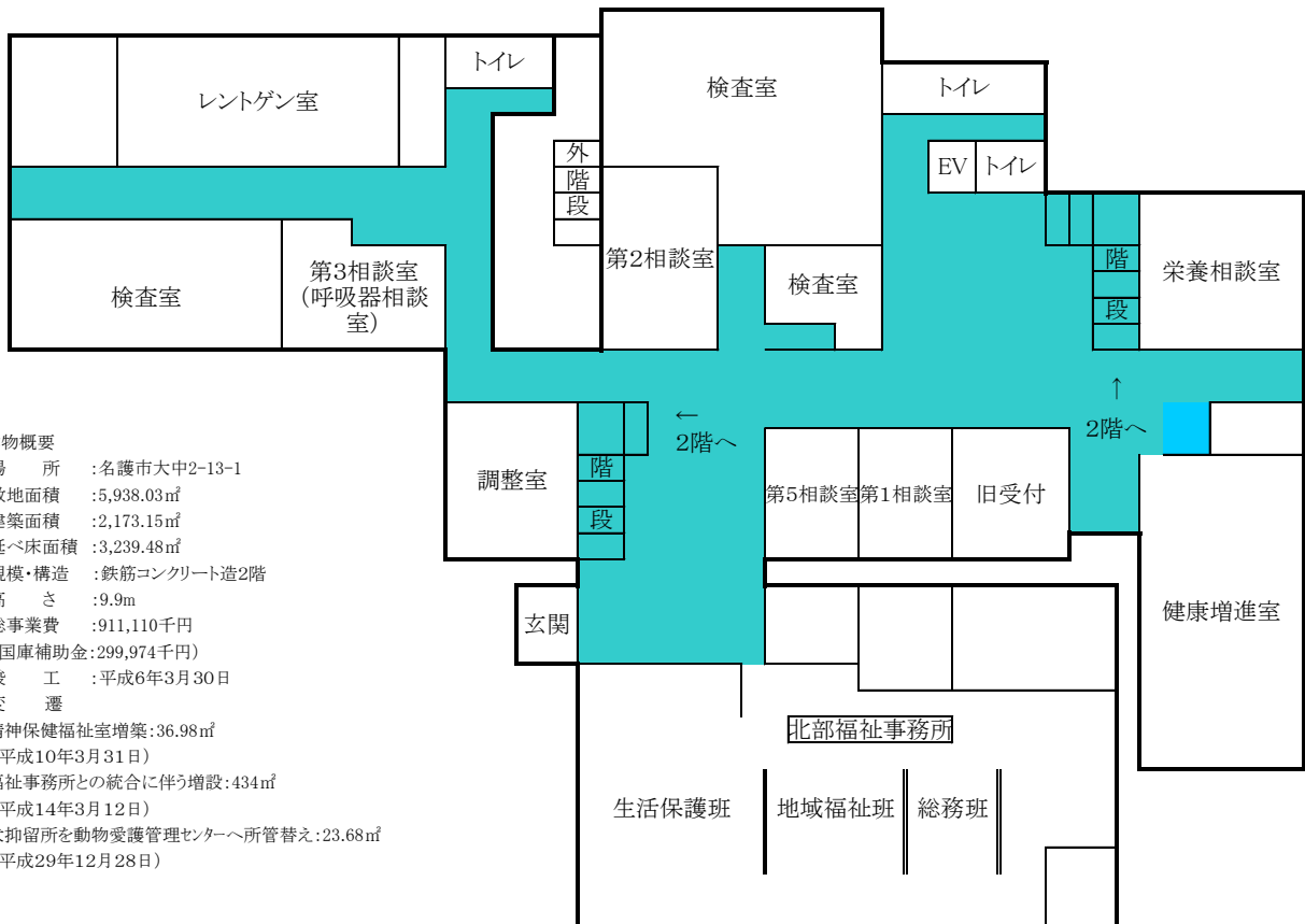
1階平面図
