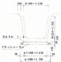
U型水路
