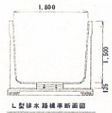
L型排水路断面図
