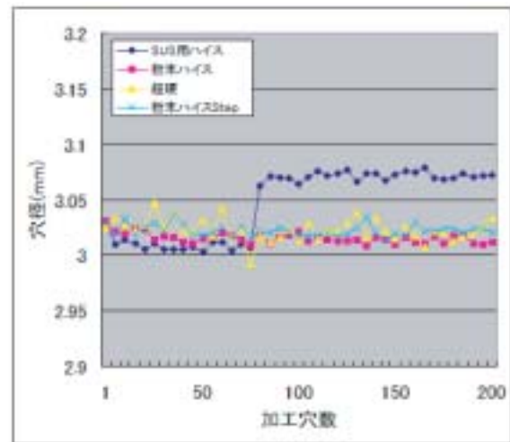
図7 加工穴数と穴径変化(SUS430)
