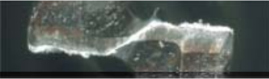
(d) 粉末ハイス Step 加工(切削速度 10m/min)
