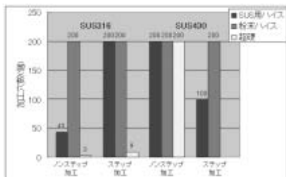
図10 工具寿命
