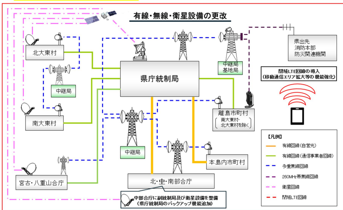
ネットワーク構成図（工事概要）
