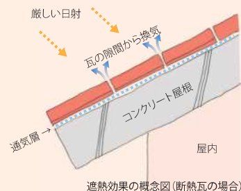
遮熱効果の概念図(断熱瓦の場合)
