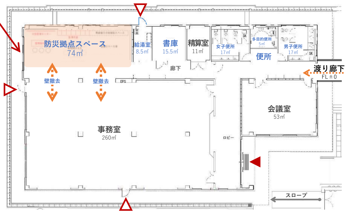
既存棟 1階平面図 (案)
