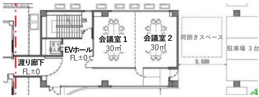
1階 平面図(案)
