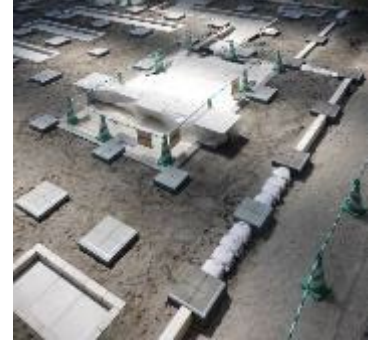
■素屋根見学エリア1階フロア【県産(与那国町)の礎石・礎盤の据え付け】
