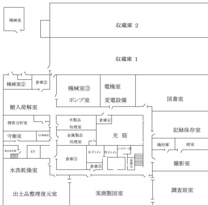
1 階平面図
