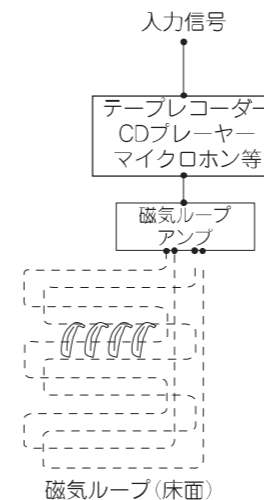
磁気ループ (聴覚障害者用集団補聴システム例)
