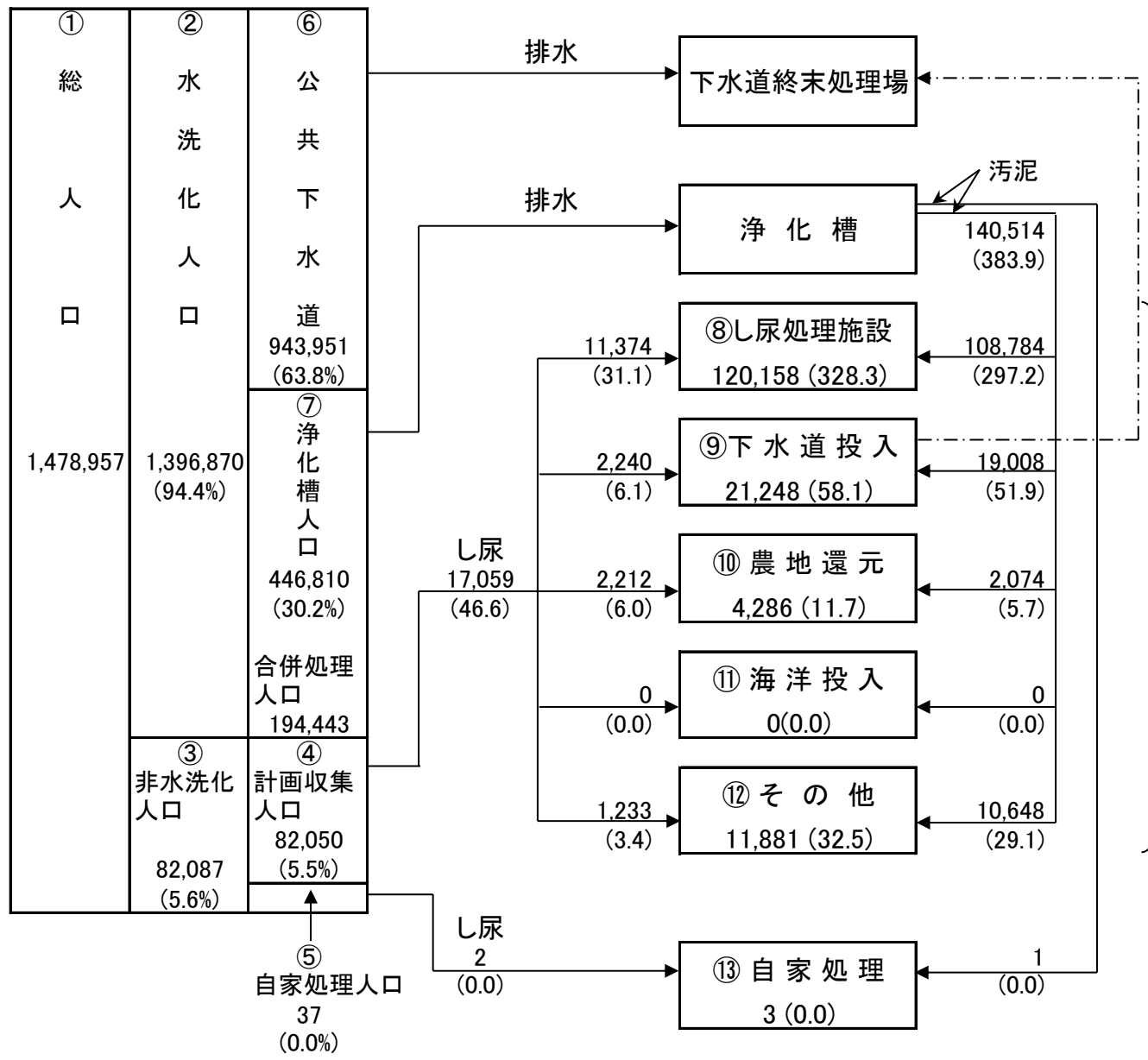
図2-9 し尿処理フローシート・し尿処理の状況(令和元年度)
