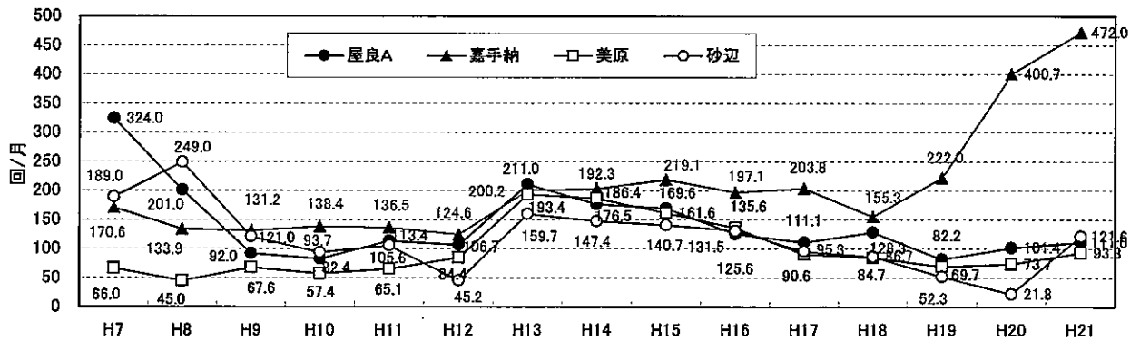
図K9-2 航空機騒音規制措置合意前後の航空機騒音発生状況 (騒音発生回数の年度推移、夜間(22時)～早朝(7時))
