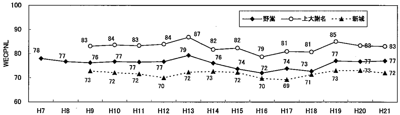
図F9 航空機騒音規制措置合意前後の航空機騒音発生状況 (WECPNLの年度推移)
