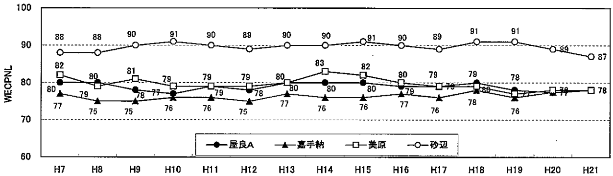
図K9 航空機騒音規制措置合意前後の航空機騒音発生状況 (WECPNLの年度推移)
