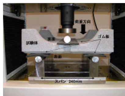
曲げ強度(破壊荷重)測定
