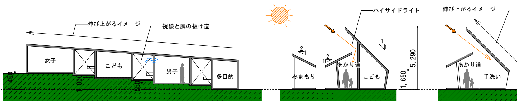
断面図 S=1/200
