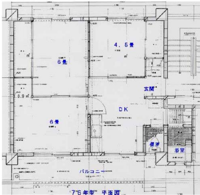
14~17棟 平面図
