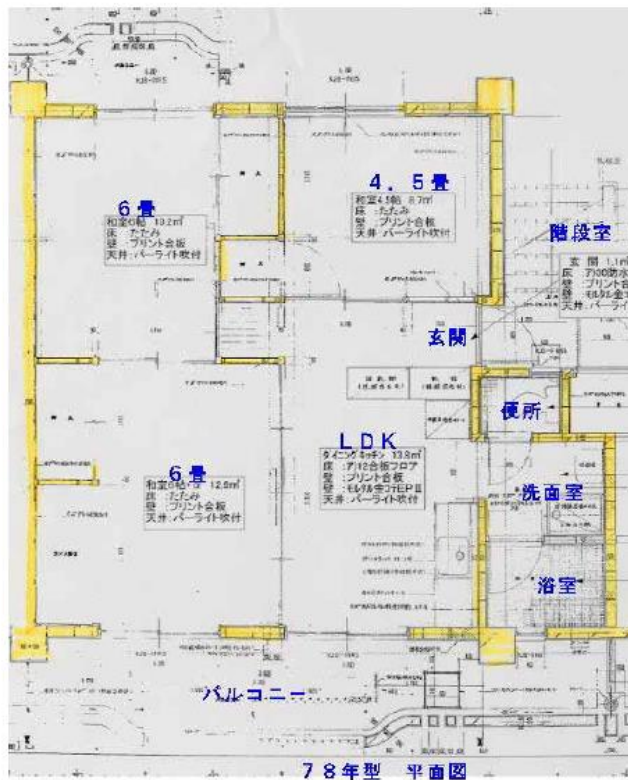
18~22棟 平面図
