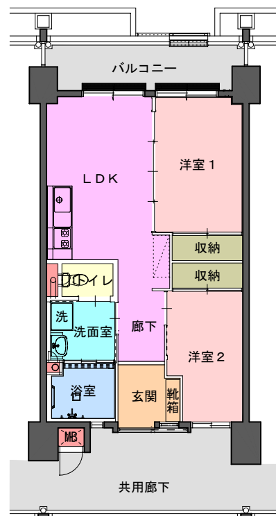
2LDK Dタイプ S=1:150
