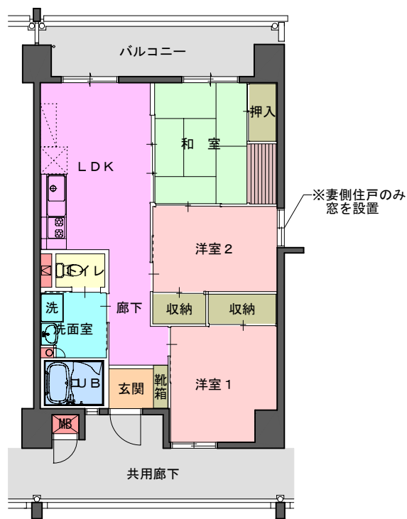
3LDK Aタイプ S=1:150
