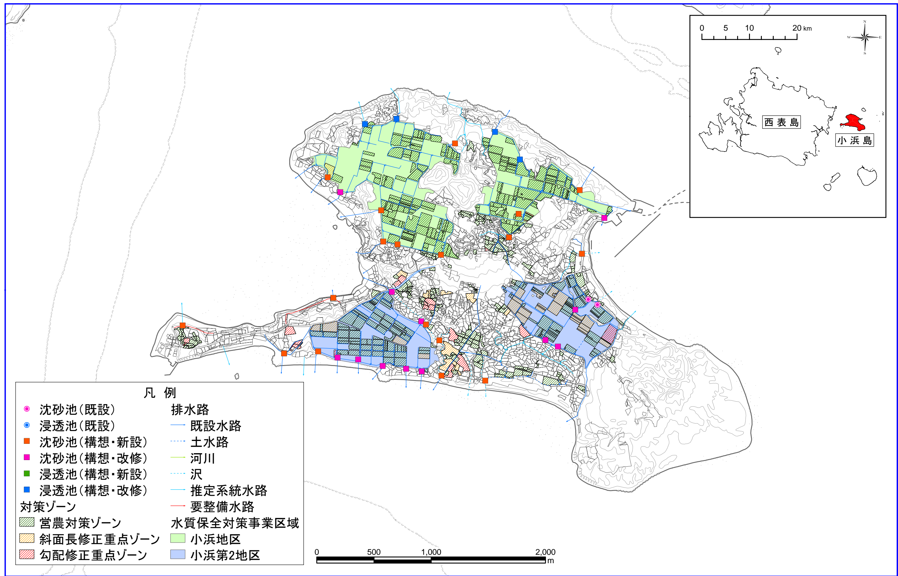
図2-27 竹富町小浜島水質保全対策事業地区設定(案)
