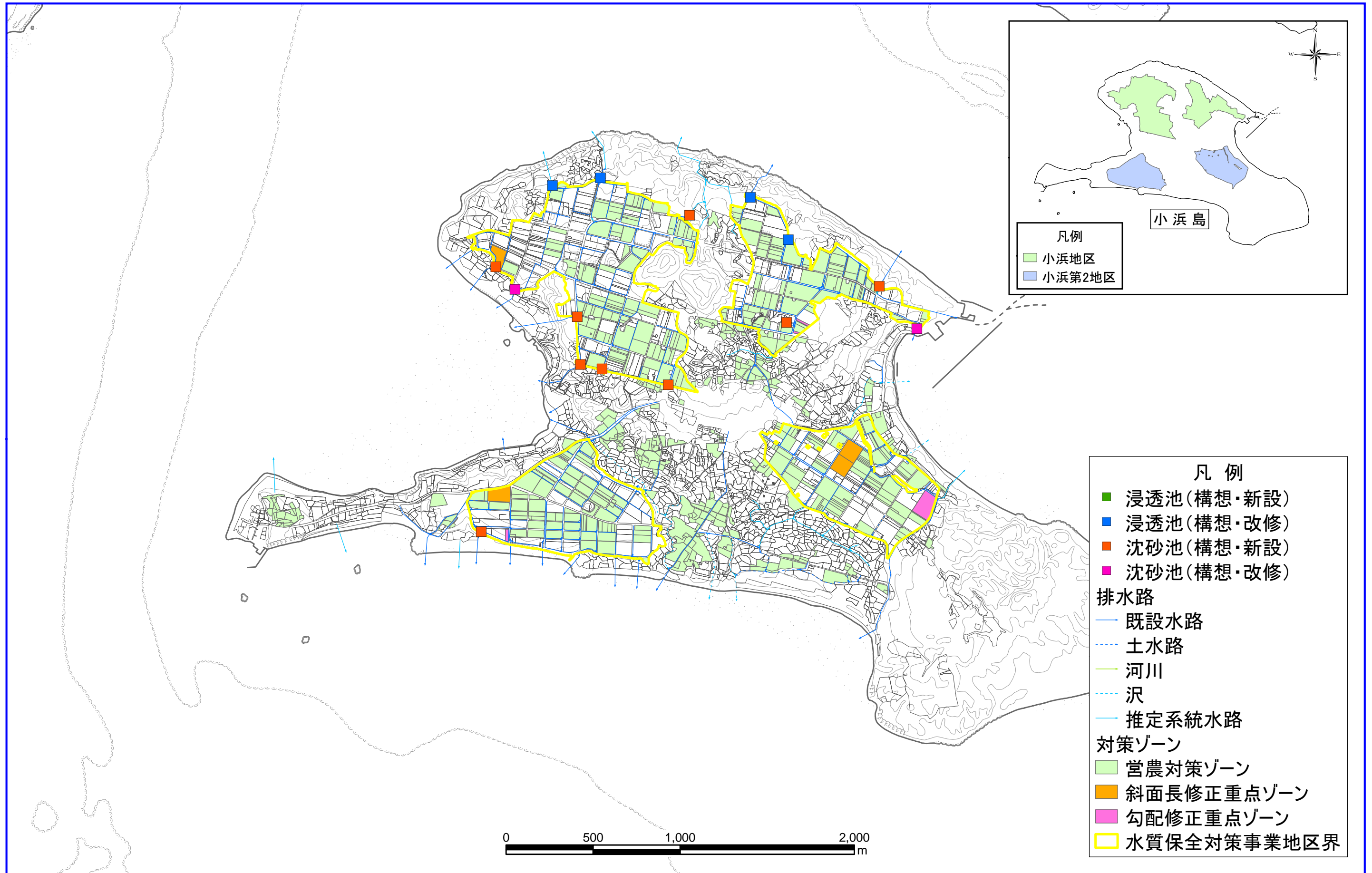
図2-30 竹富町小浜島地域が一体となった効率的かつ持続的な(H27年度目標)赤土等流出対策構想図
