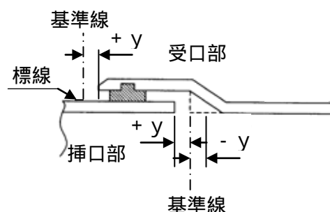
T形
